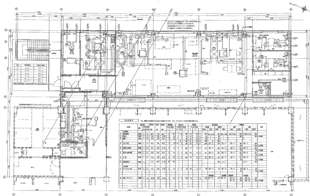
2階平面図・S=1/200 (空調設備 増築後)
